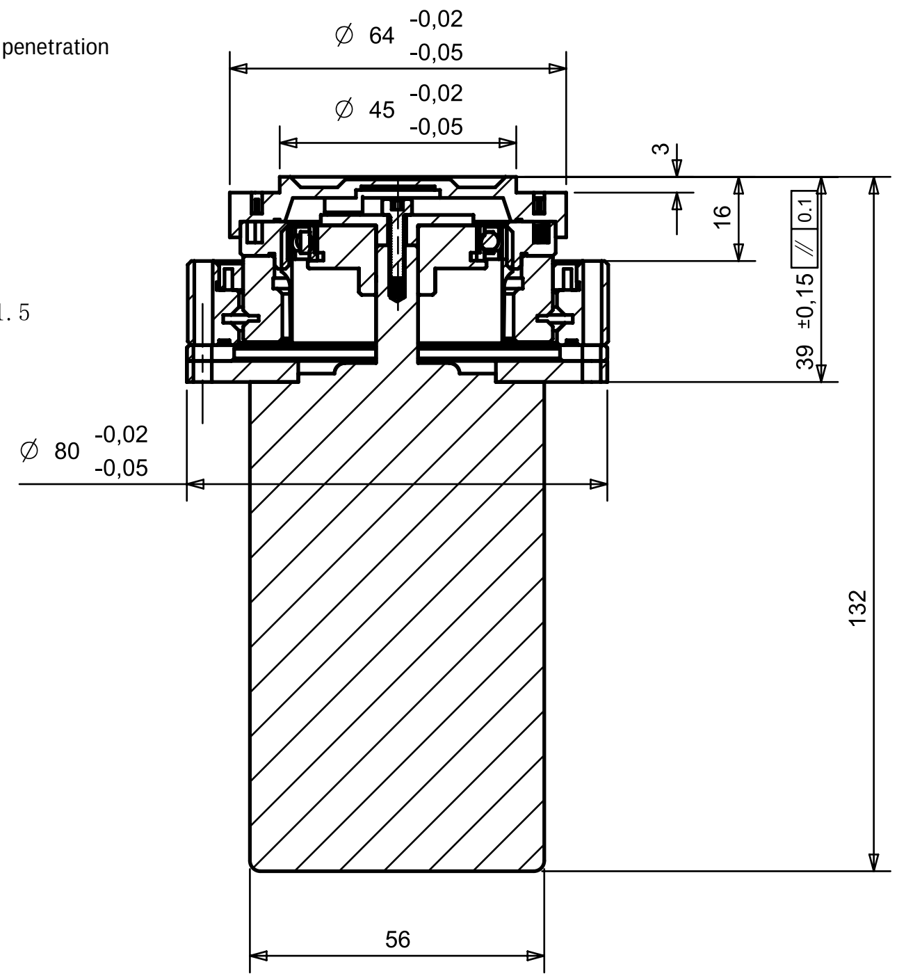
SECTION A-A
